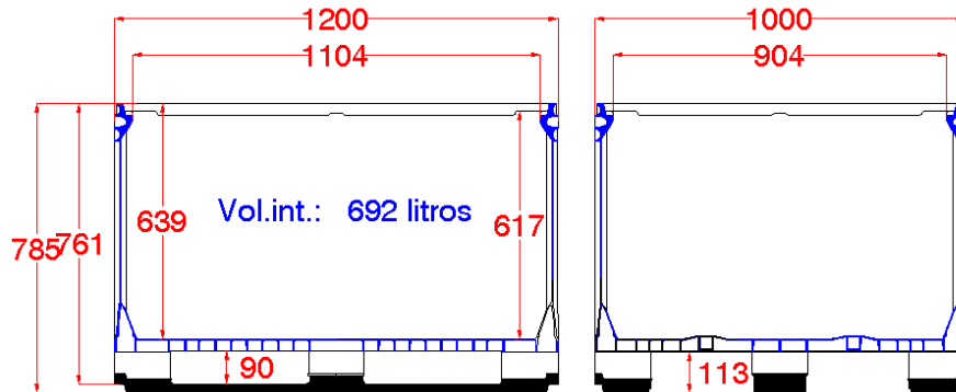
Palox 1200 x 1000 x 785, fond et parois ajourés, 3 semelles
